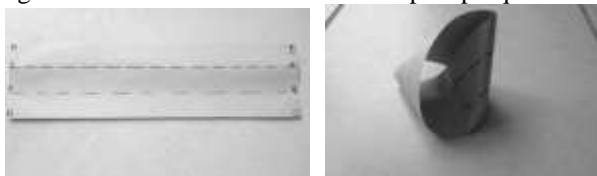
Figura 8-Faixa de Möebius construída pela pesquisadora.
