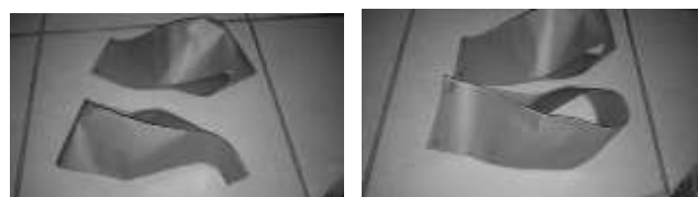
Figura 12-Faixas de Möebius obtidas a partir do corte da Garrafa de Klein. Foto da pesquisadora.
