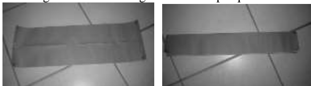
Figura 10-Tira retangular. Foto da pesquisadora.
