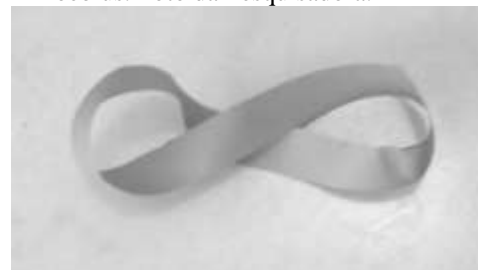
Figura 7- Superfície obtida após o recorte da faixa de Möebius. Foto da Pesquisadora.
