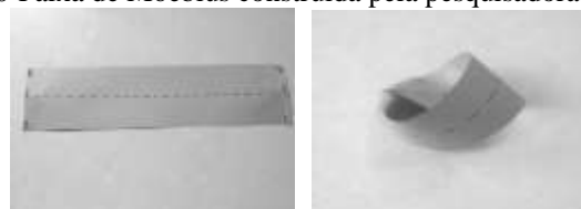
Figura 6-Faixa de Möebius construída pela pesquisadora.
